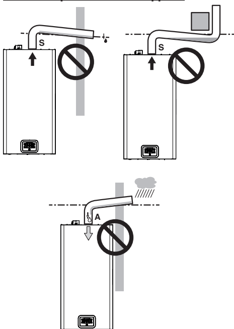
Figura 5.7 A = aspirazione aria S = scarico fumi
